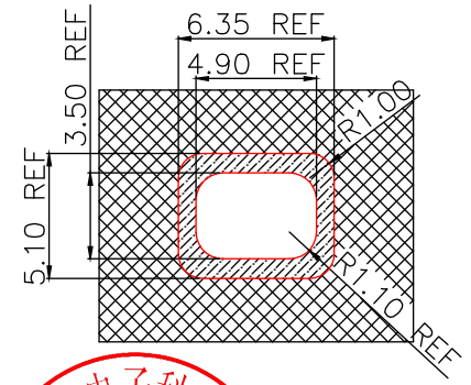
面板开孔参考尺寸
